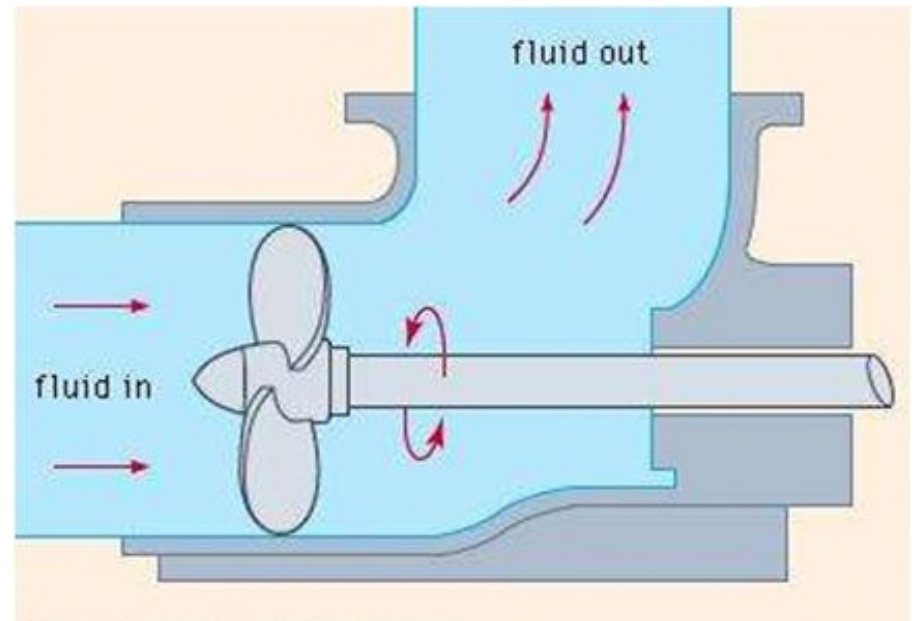
Pompa assiale
