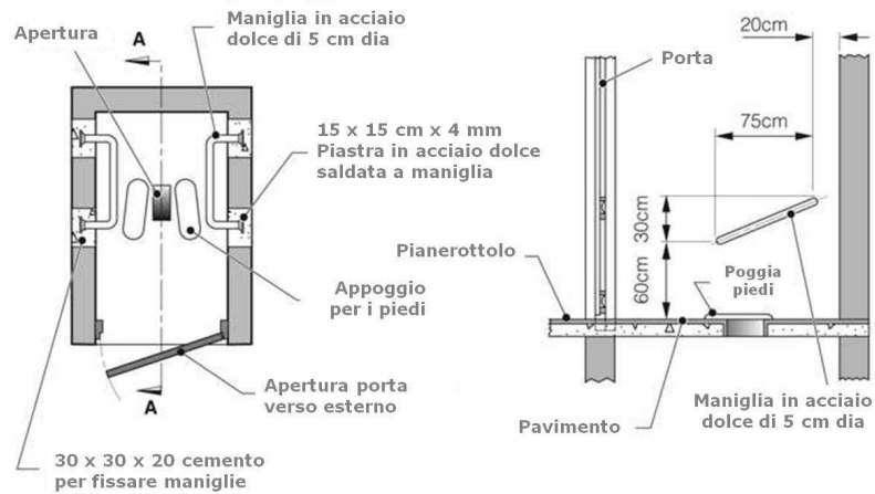
Sezione di A-A
