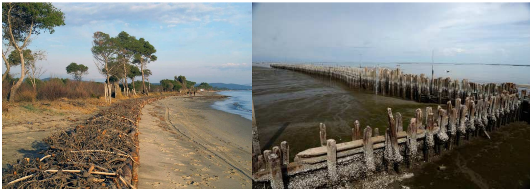
Barriere rivierasche antierosione in aree soggette ad uragani
