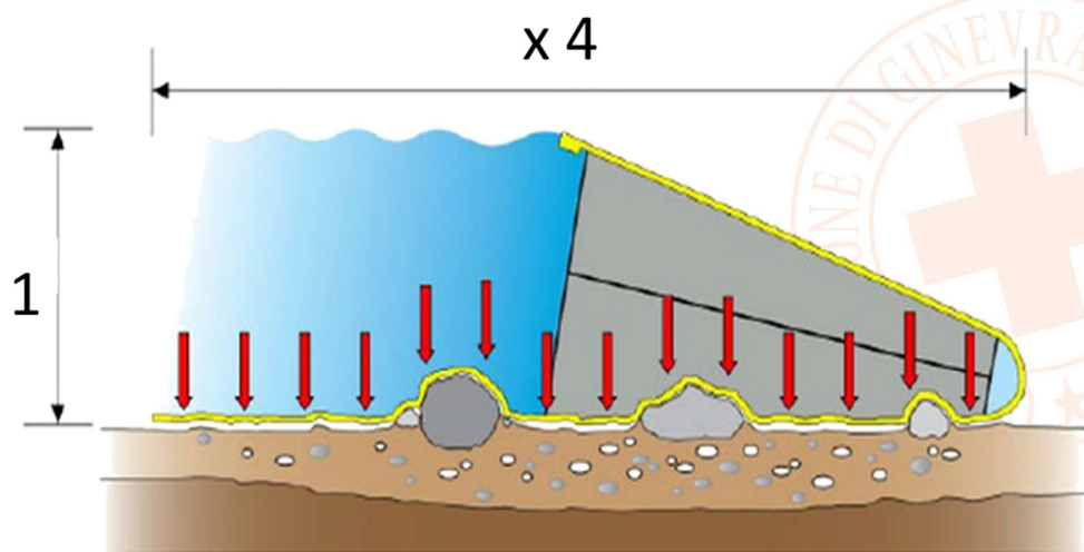
Come funziona una barriera passiva antiallagamento
